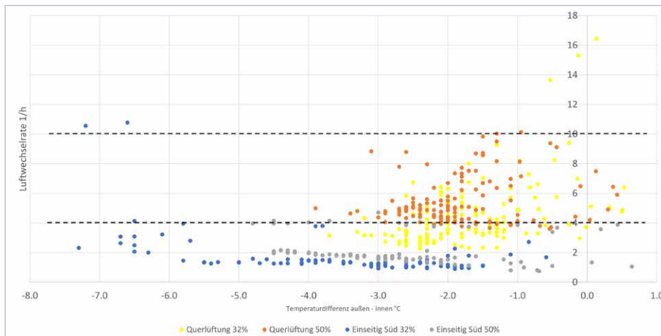
Luftwechselraten in Abhängigkeit der Temperaturdifferenz bei einseitiger Lüftung & Querlüftung
